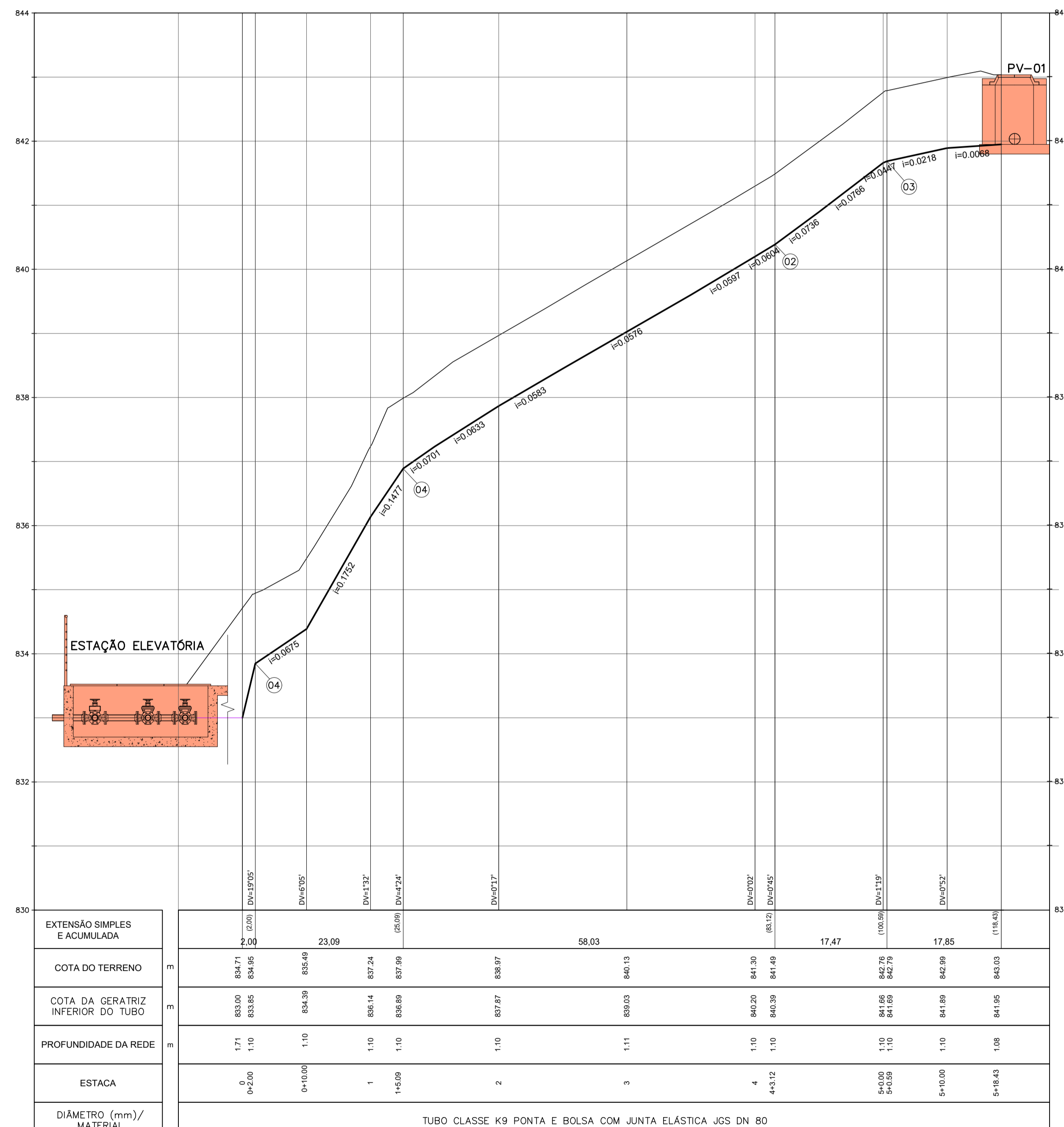
PERFIL ESC.: H=1:500 V=1:50
