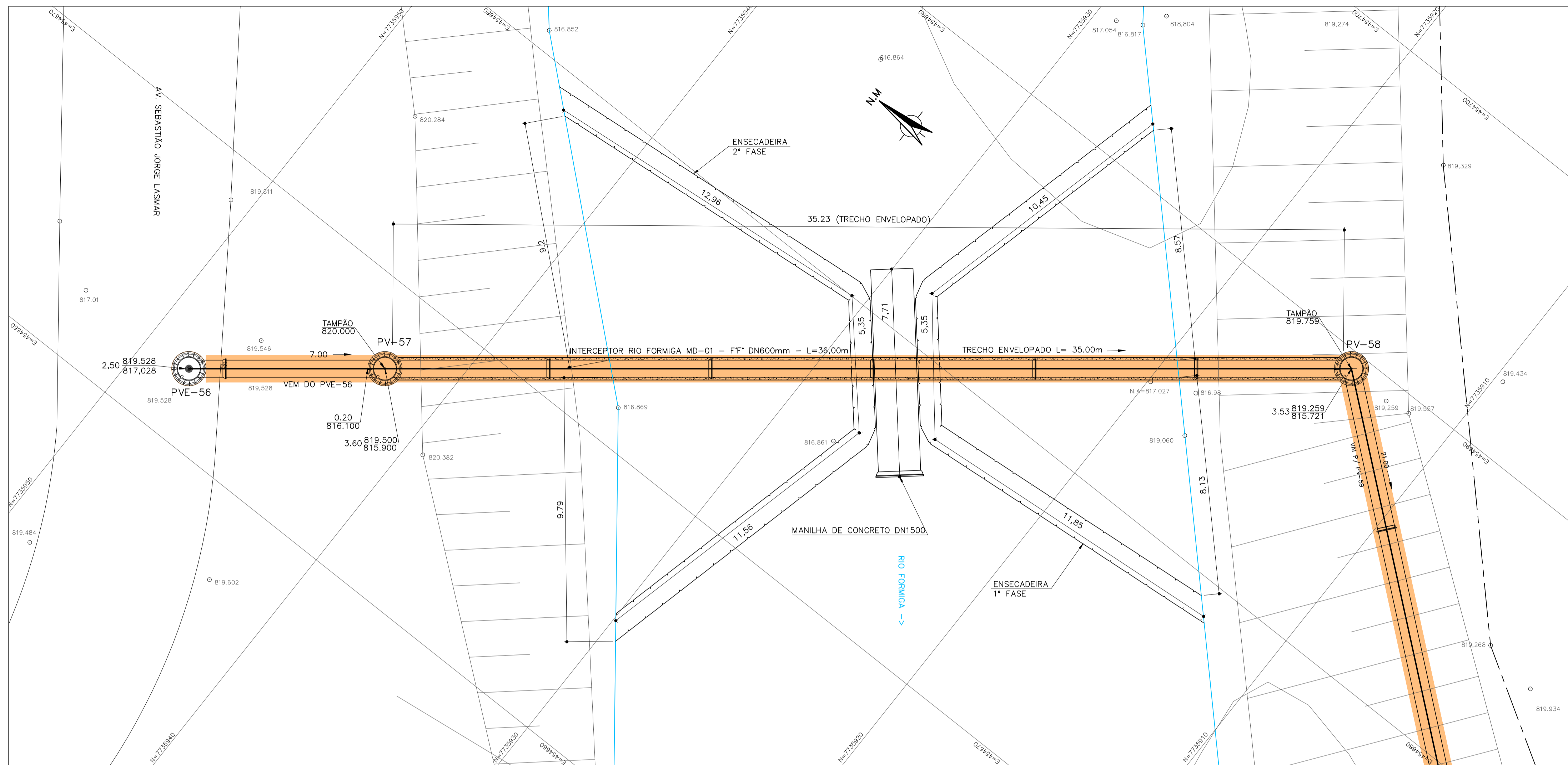
PLANTA ESC.: 1:100
