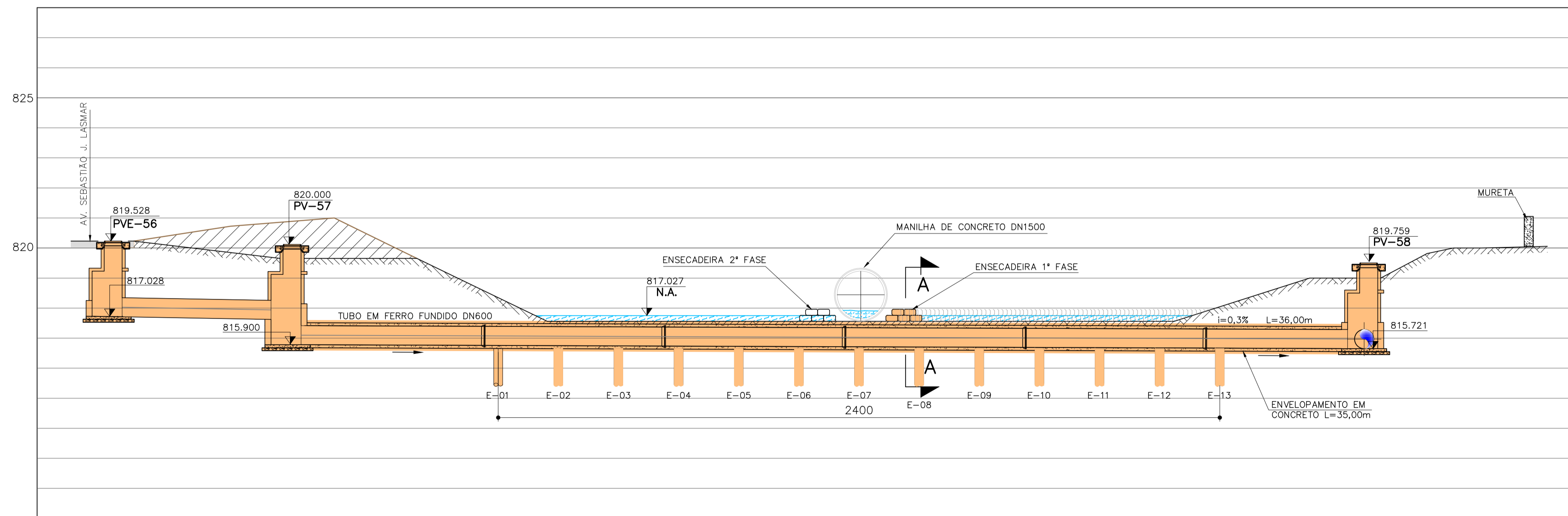
PERFIL ESC.: 1:100
