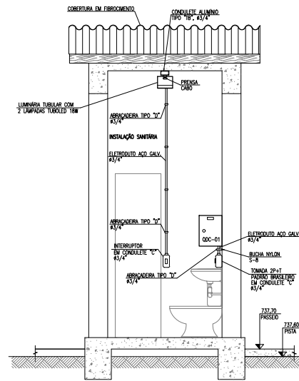
BANHEIRO - ILUMINAÇÃO E TOMADAS - CORTE AA ESC:1:25
