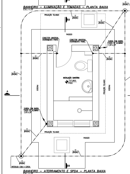
BANHEIRO - ATERRAMENTO E SPDA - PLANTA BAIXA ESC:1:25
