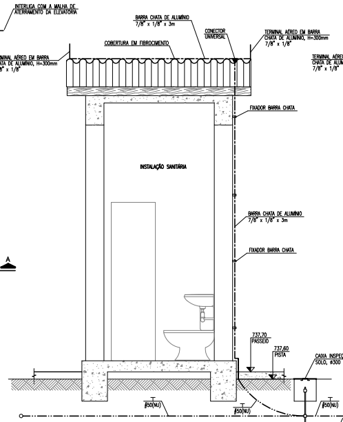
BANHEIRO - ATERRAMENTO E SPDA - CORTE AA ESC:1:25
