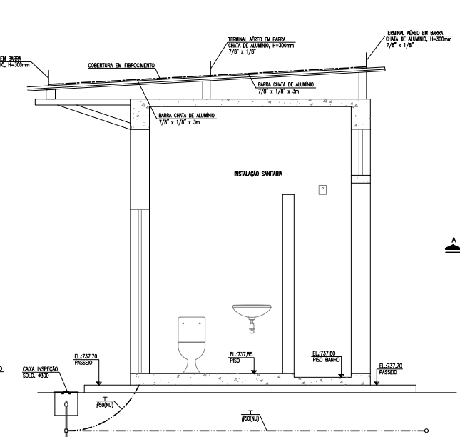
BANHEIRO - ATERRAMENTO E SPDA - CORTE BB ESC:1:25
