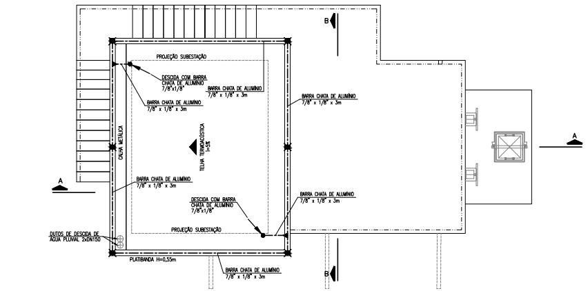
ELEVATÓRIA - ATERRAMENTO E SPDA - COBERTURA ESCALA: 1:50
