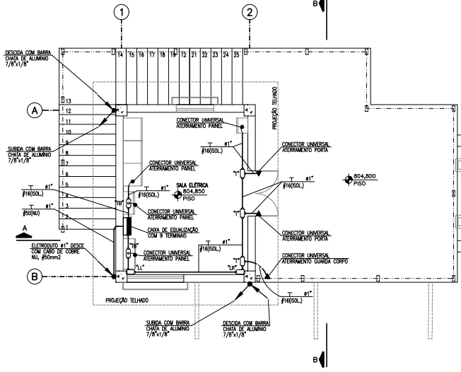
ELEVATÓRIA - ATERRAMENTO E SPDA - EL. 810.00 - PLANTA BAIXA ESCALA: 1:50
