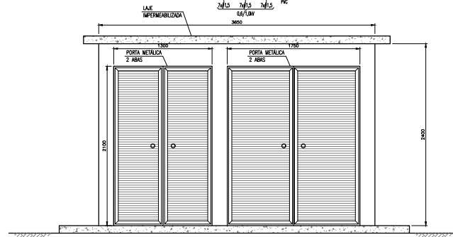
ABRIGO ELÉTRICO - VISTA A ESC: 1:25
