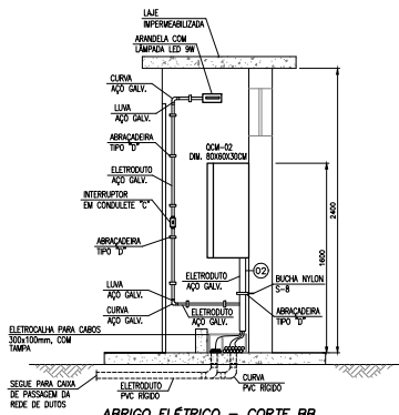
ABRIGO ELÉTRICO - CORTE BB ESC: 1:25
