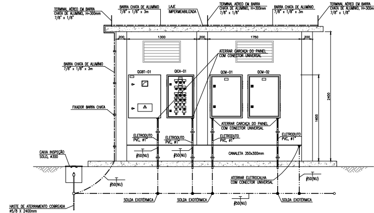
ABRIGO ELÉTRICO - CORTE CC ESC: 1:25
