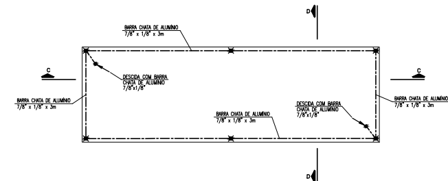
ABRIGO ELÉTRICO - MALHA DE CAPTAÇÃO - COBERTURA ESC: 1:25
