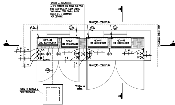
ABRIGO ELÉTRICO - ILUMINAÇÃO - TOMADAS - FORÇA - PLANTA BAIXA ESC: 1:25
