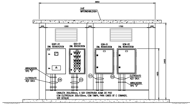
ABRIGO ELÉTRICO - CORTE AA ESC: 1:25
