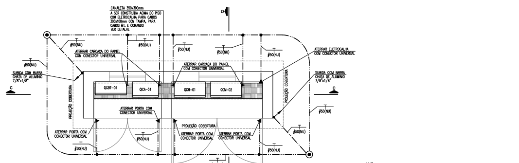
ABRIGO ELÉTRICO - MALHA DE ATERRAMENTO - PLANTA BAIXA ESC: 1:25
