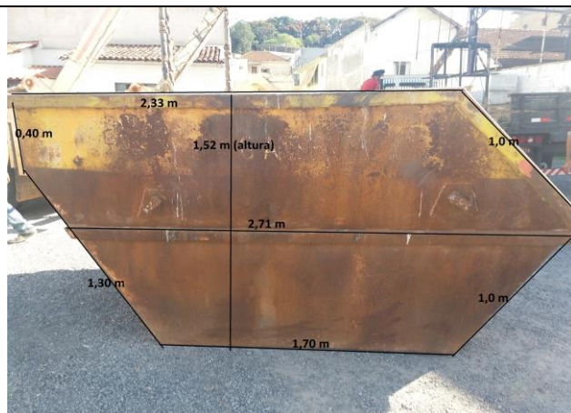
Foto 01: Vista Lateral.
